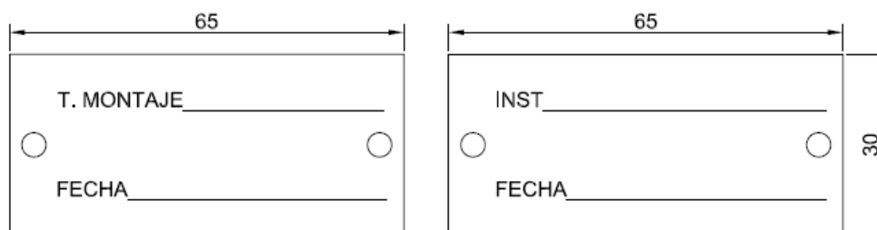
Figura 21. Placa fijación embarrado.
