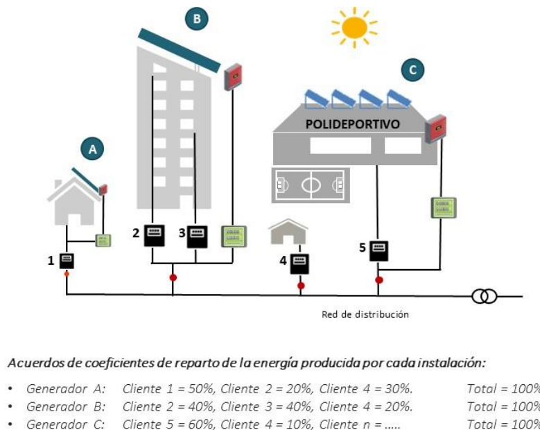
FIGURA C.11. Autoconsumo COLECTIVO con generación en RED INTERIOR y A TRAVÉS de red con repartos separados por generación
